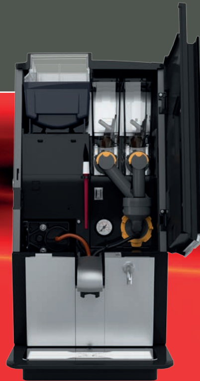
Esprecious 22 mit geteiltem Bohnenbehälter und 2 Instantbehältern
