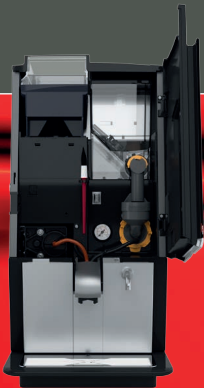
Esprecious 11 mit 1 Bohnenbehälter und 1 Instantbehälter
