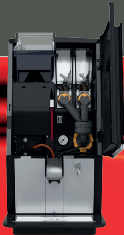
Esprecious 12 mit 1 Bohnenbehälter und 2 Instantbehältern
